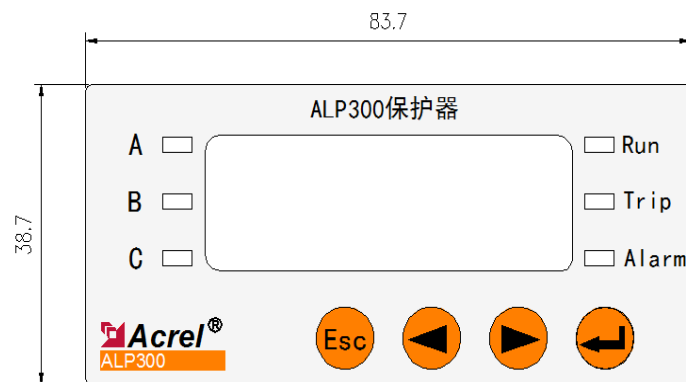
主视图 Front view
